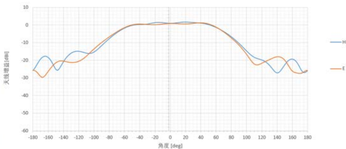
图 8 系统方向图
