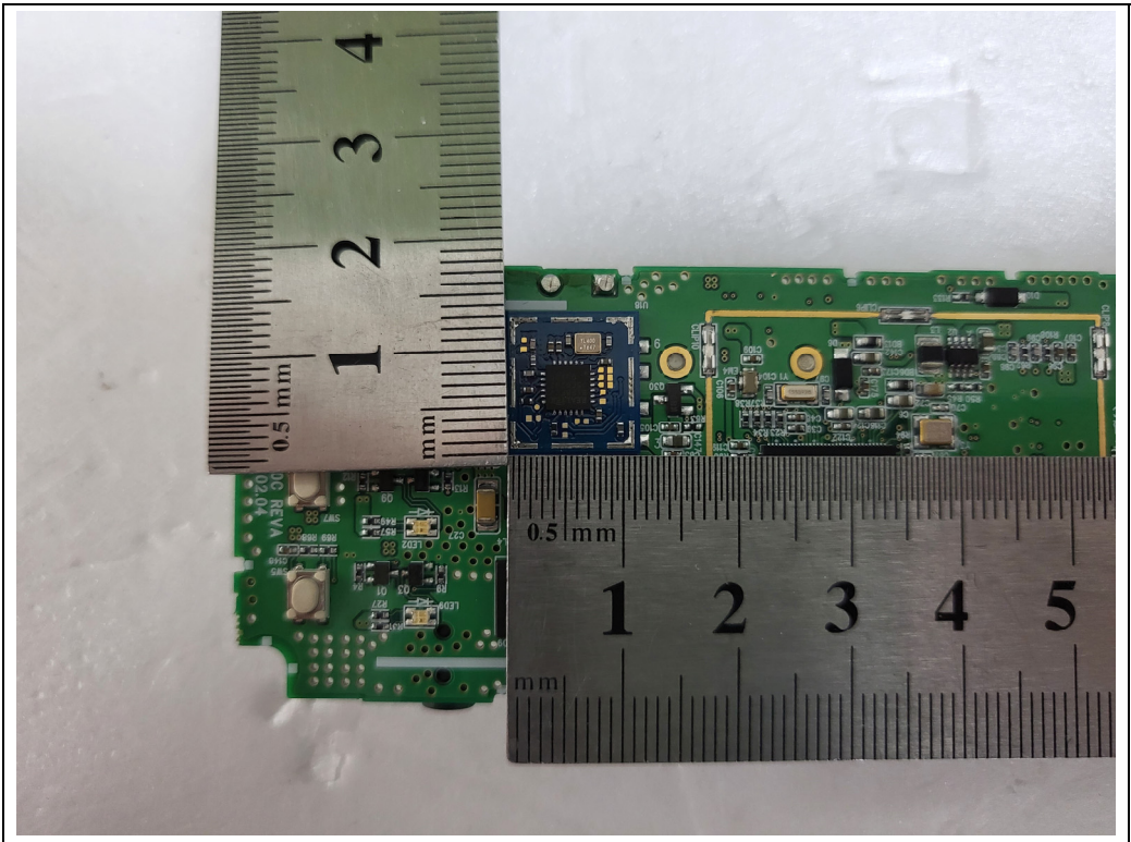
<Wifi Module>
