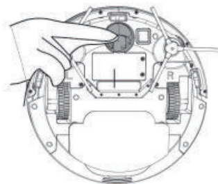
b. Nettoyage de la roue motrice et de la roue universelle
