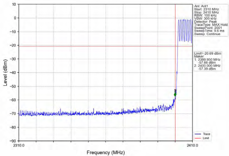
GFSK_DH5_HOPP_2410MHz_Ant1_NTNV
