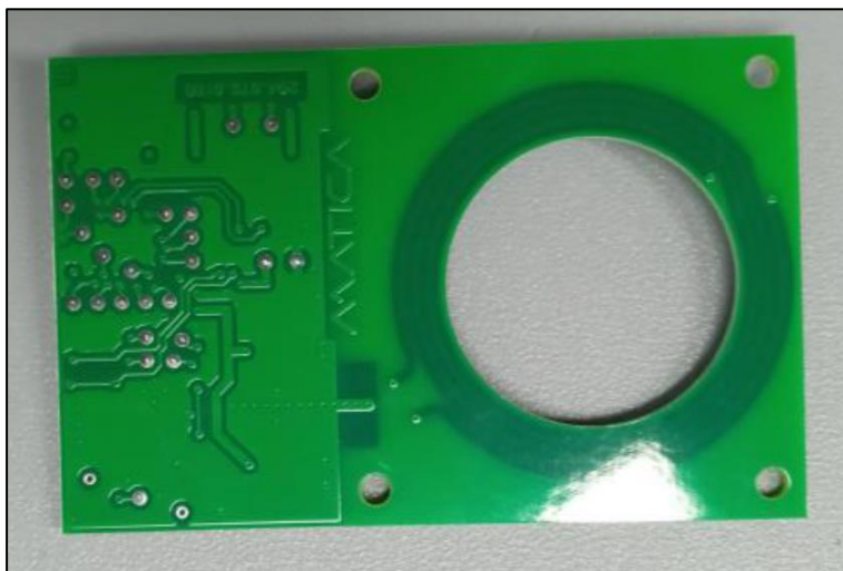
RFID PCBA
