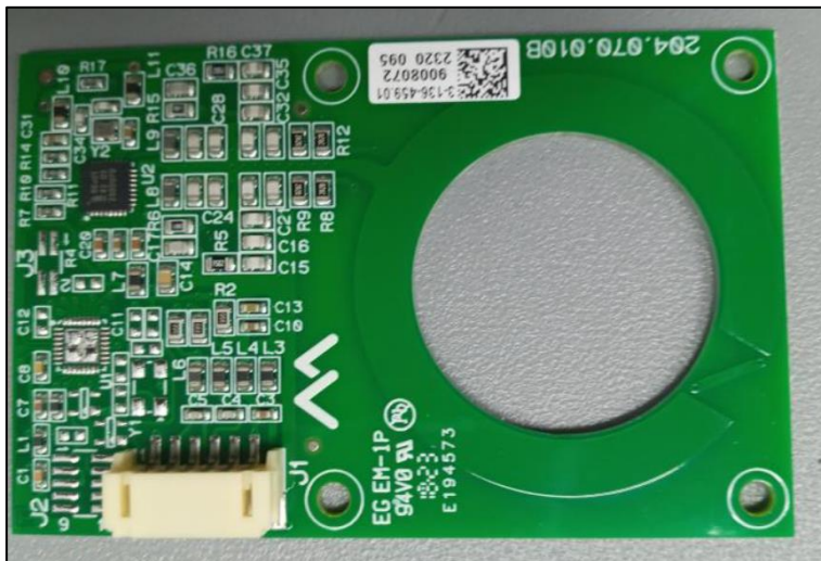
RFID PCBA
