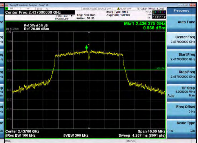
802.11n(HT20) CH06
