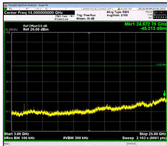
3GHz-25GHz
