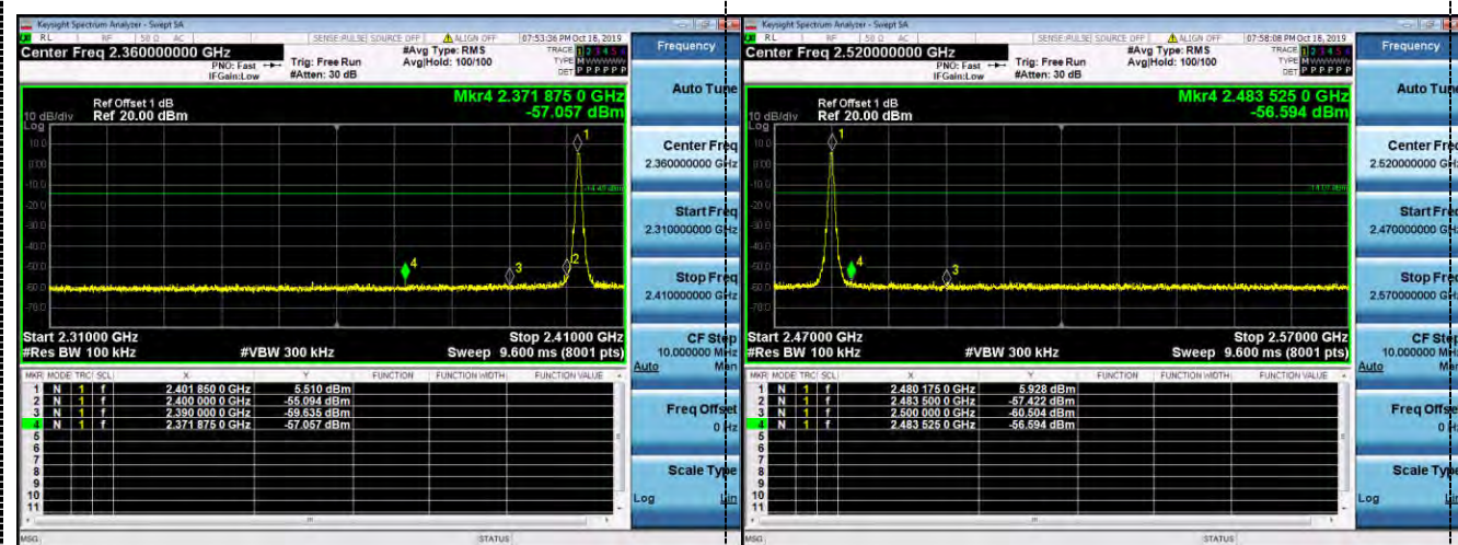
Left Band edge hoping off
