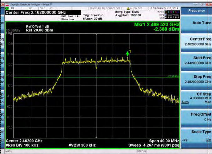
802.11g CH11
