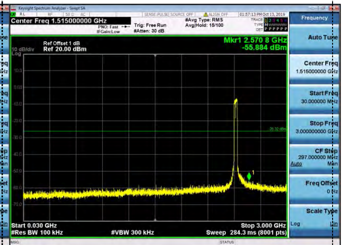
30MHz-3GHz
