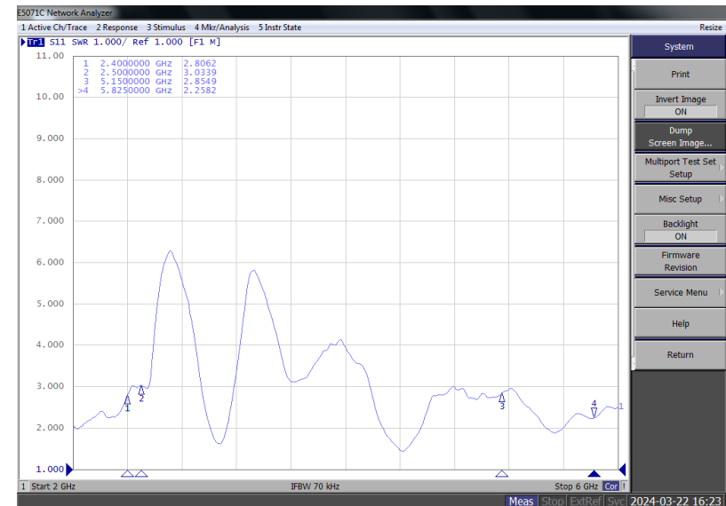
VSWR
