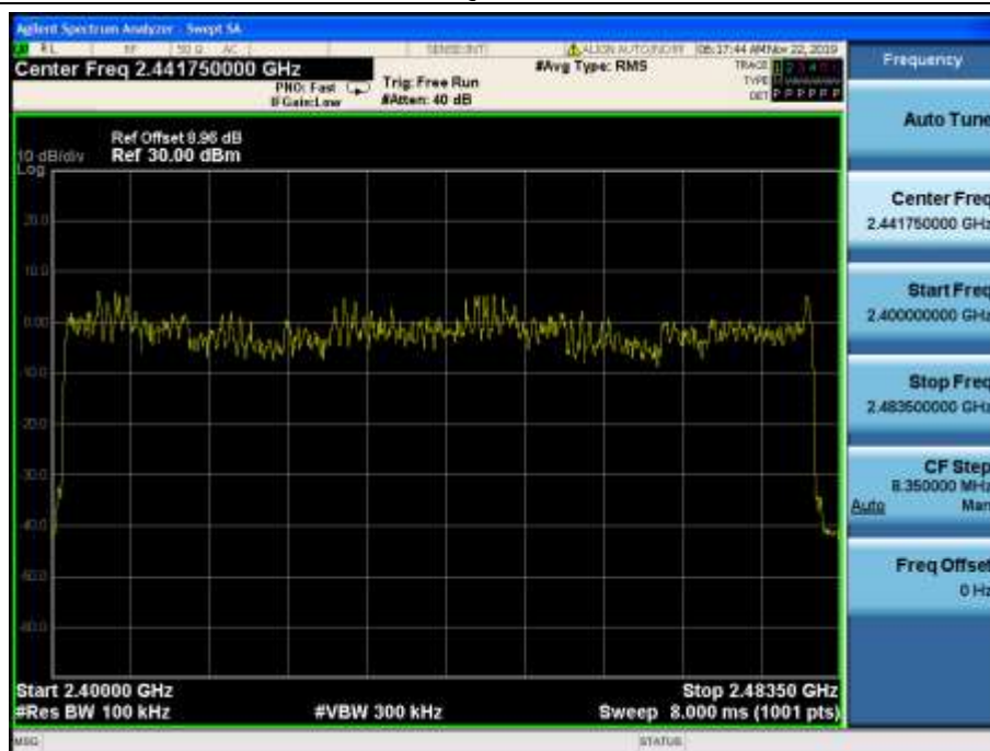
\pi/4 -DQPSK mode
