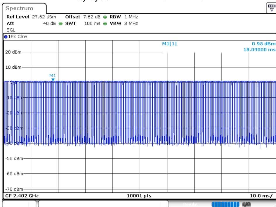
Duty Cycle NVNT BLE 2402MHz Ant 1
