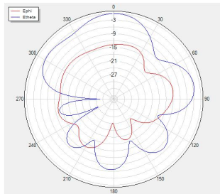
Theta=90 freq=1720MHz
