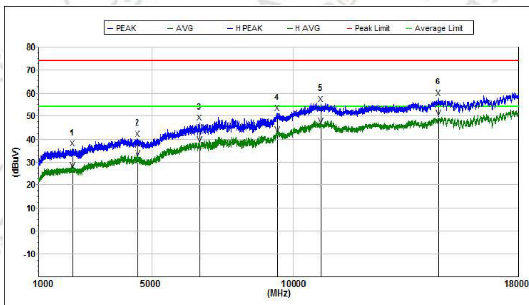
802.11b 2412 Horizontal
