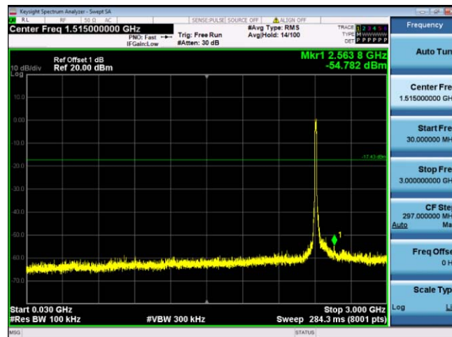
30MHz-3GHz
