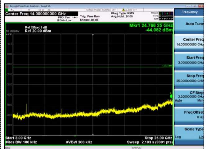
3GHz-25GHz
