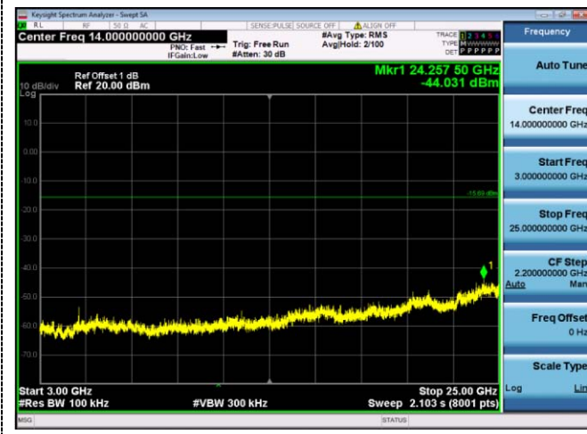
3GHz-25GHz
