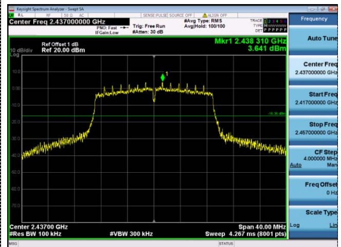
802.11n(HT20) CH06
