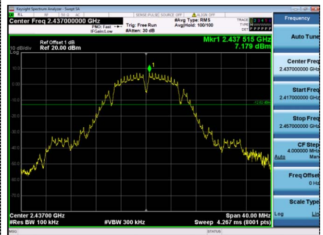
802.11b CH06
