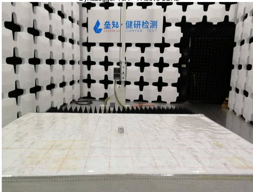
DynaLogger TcA+ : Above 1GHz
