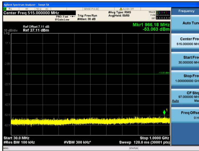
Band2-3MHz-QPSK-18615-1RB#0-30~1000MHz
