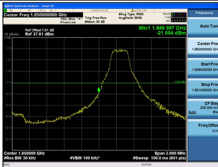
Band2-3MHz-QPSK-18615-1RB#0
