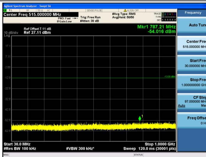
Band2-3MHz-QPSK-18900-1RB#0-30~1000MHz
