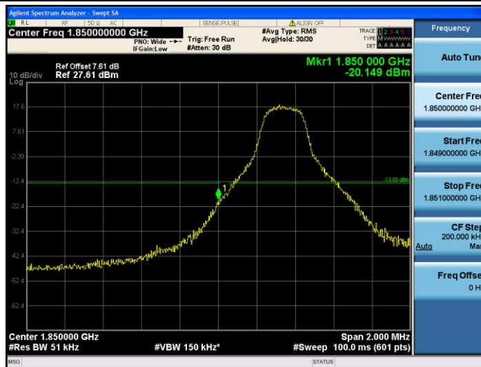
Band2-5MHz-16QAM-18625-1RB#0
