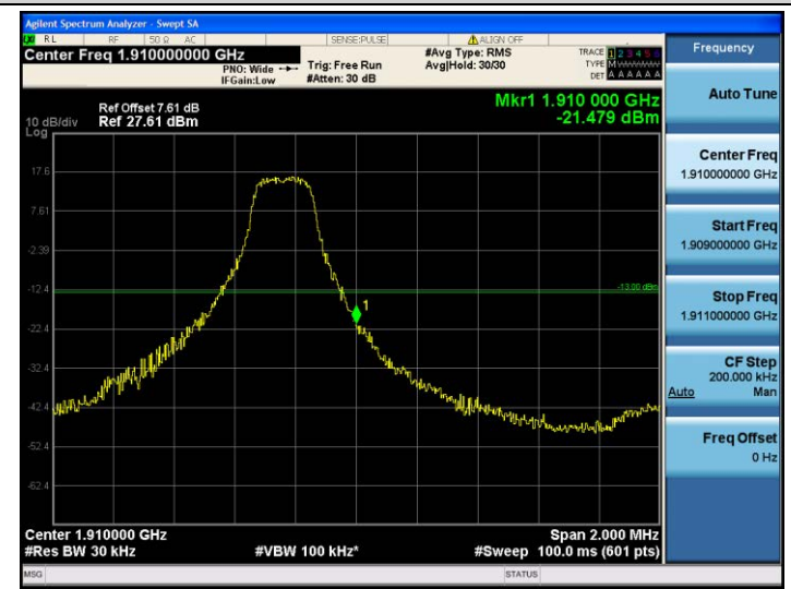
Band2-3MHz-QPSK-19185-1RB#14
