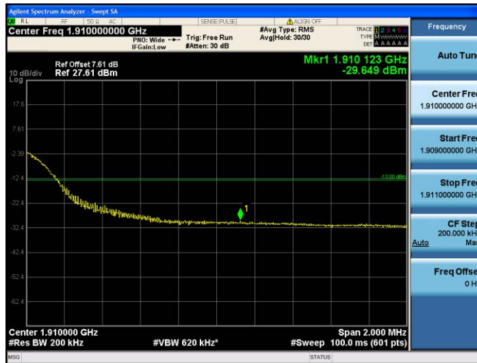
Band2-20MHz-QPSK-19100-100RB#0
