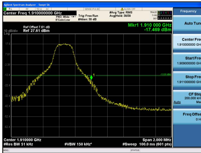
Band2-5MHz-QPSK-19175-1RB#24
