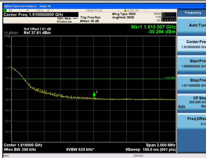
Band2-20MHz-16QAM-19100-100RB#0
