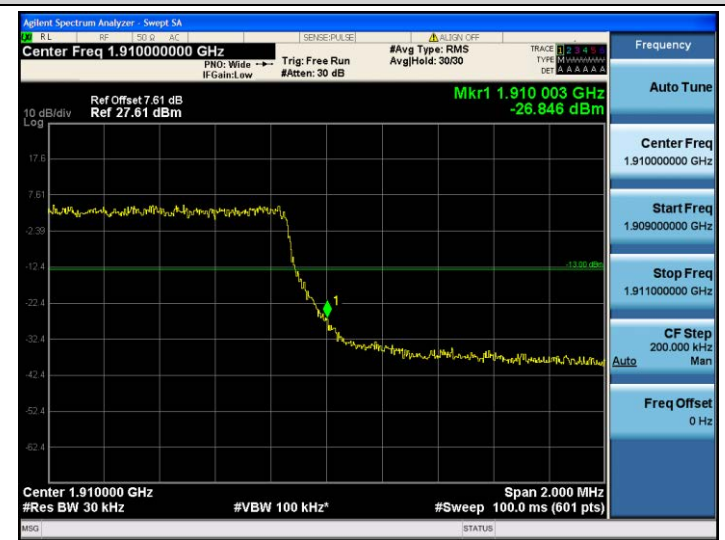
Band2-3MHz-QPSK-19185-15RB#0
