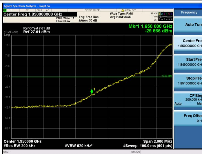
Band2-20MHz-16QAM-18700-1RB#0
