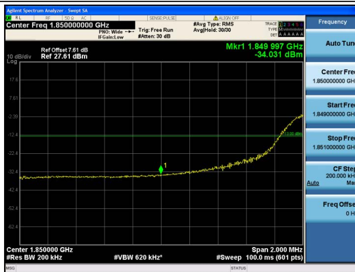
Band2-20MHz-QPSK-18700-100RB#0
