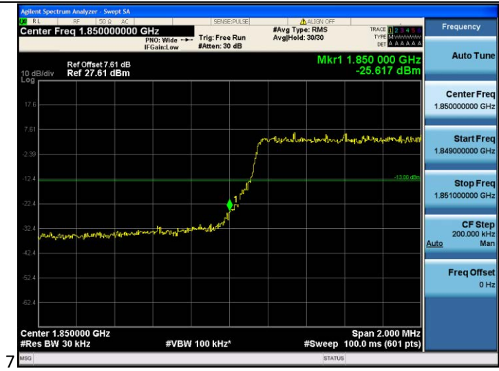
Band2-3MHz-QPSK-18615-15RB#0
