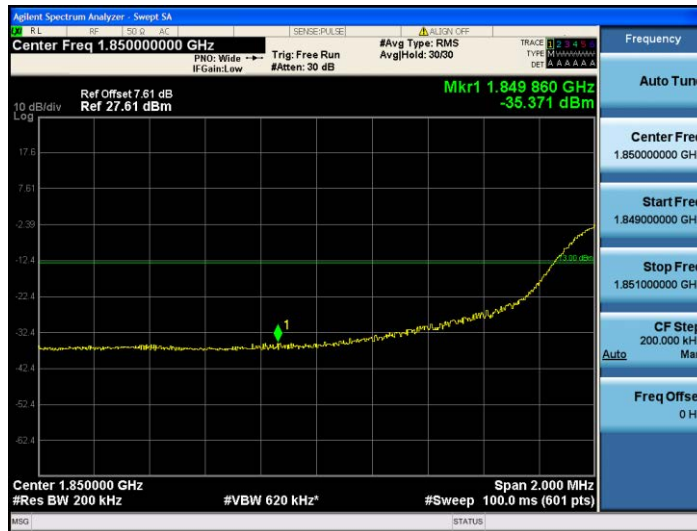
Band2-20MHz-16QAM-18700-100RB#0
