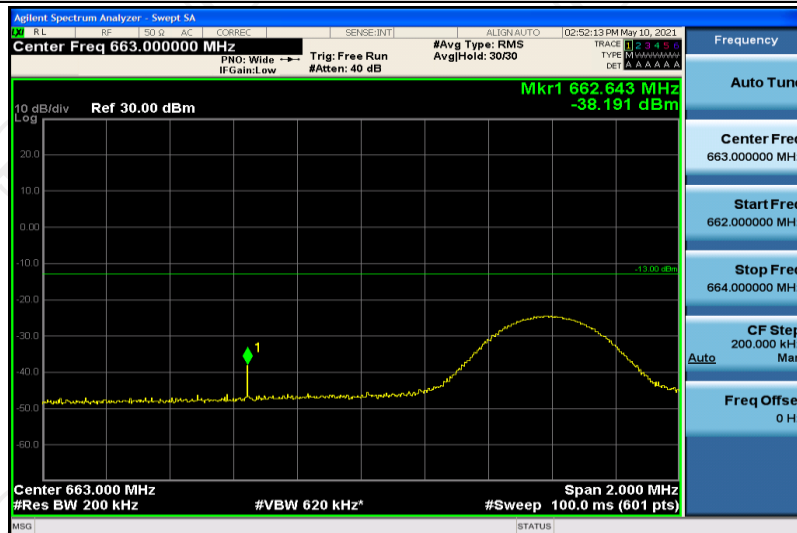
Band71-10MHz-QPSK-133172-1RB#0
