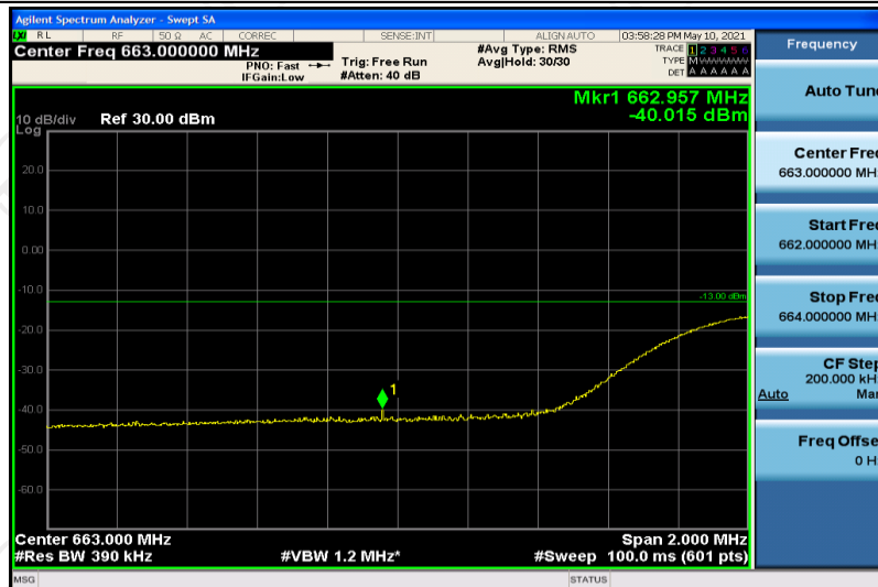
Band71-20MHz-QPSK-133222-1RB#0
