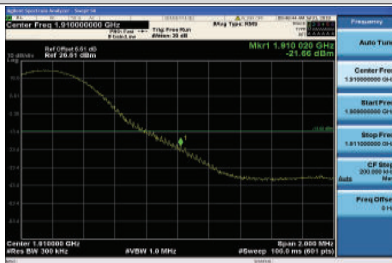
Band2-15MHz-16QAM-19125-1RB#74
