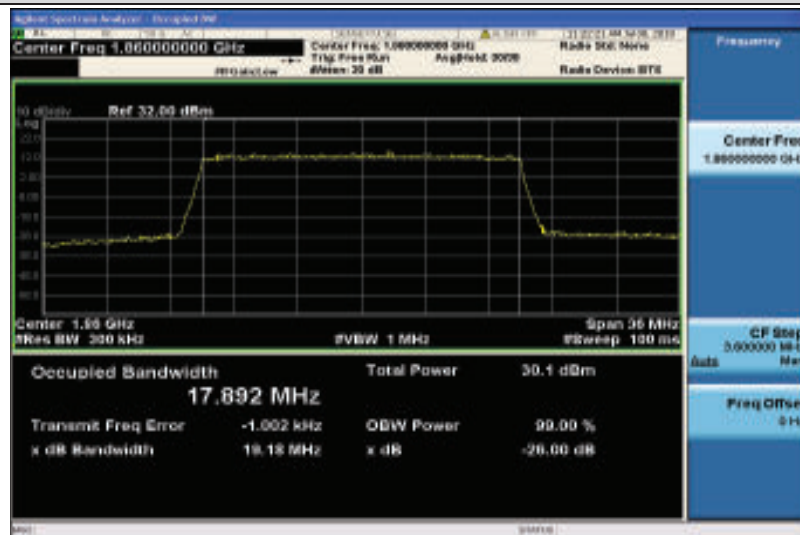
Band2-20MHz-QPSK-18700-100RB#0-17.892
