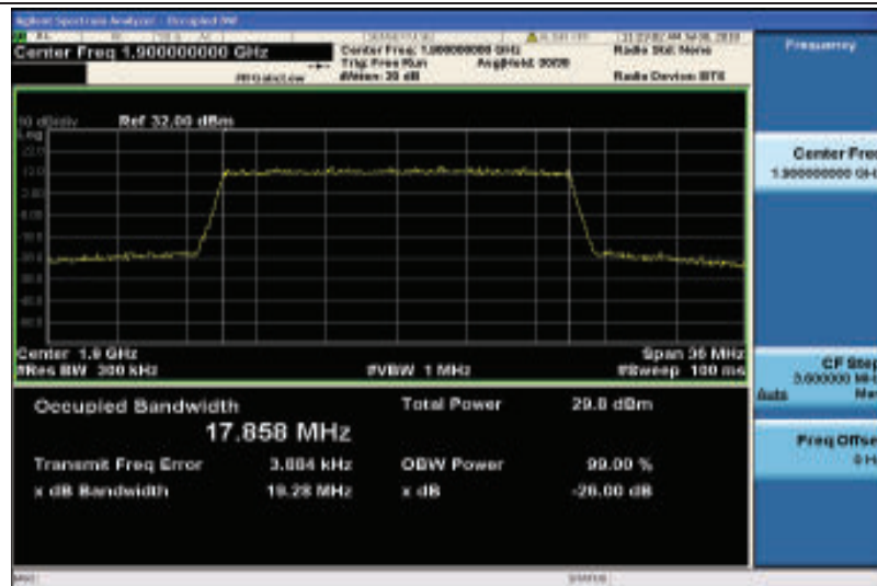
Band2-20MHz-QPSK-19100-100RB#0-17.858
