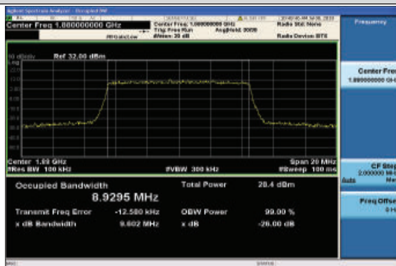
Band2-10MHz-16QAM-18900-50RB#0-8.9295
