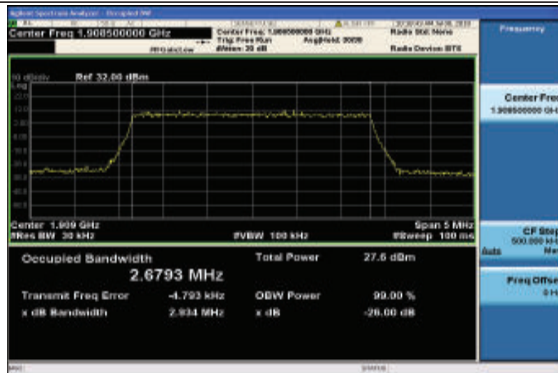
Band2-3MHz-16QAM-19185-15RB#0-2.6793
