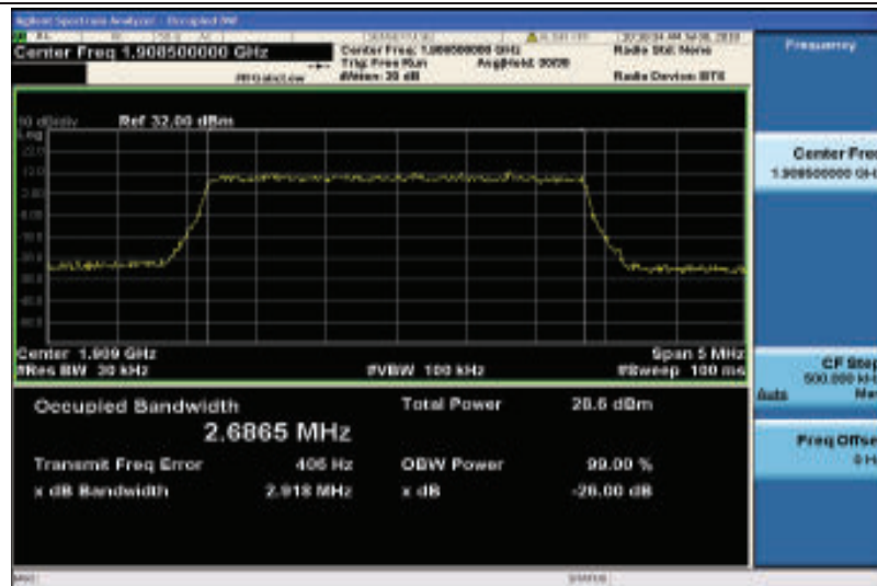
Band2-3MHz-QPSK-19185-15RB#0-2.6865
