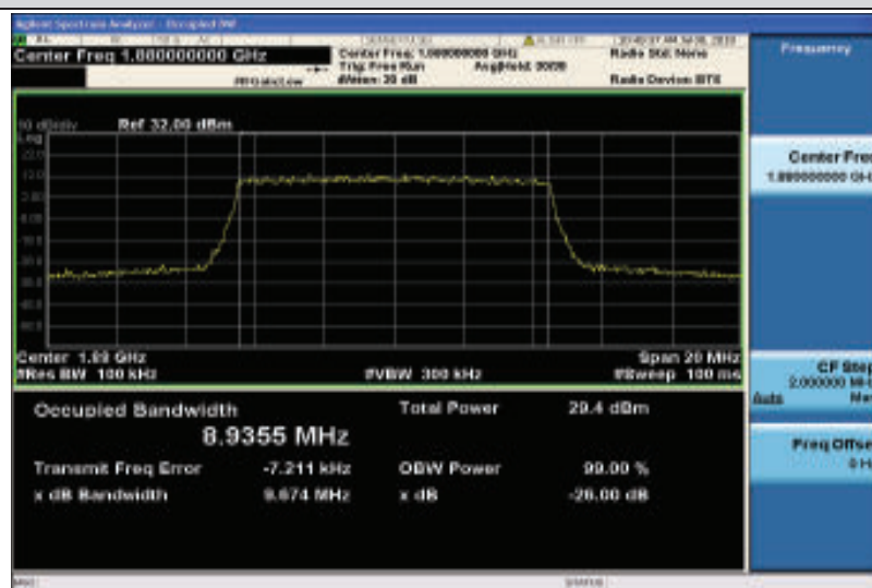
Band2-10MHz-QPSK-18900-50RB#0-8.9355
