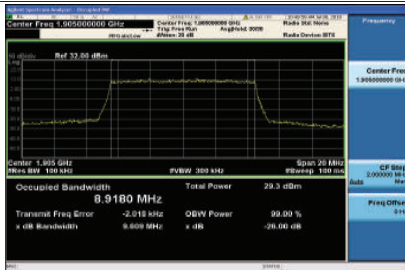
Band2-10MHz-QPSK-19150-50RB#0-8.9180
