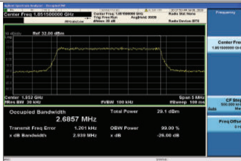
Band2-3MHz-QPSK-18615-15RB#0-2.6857
