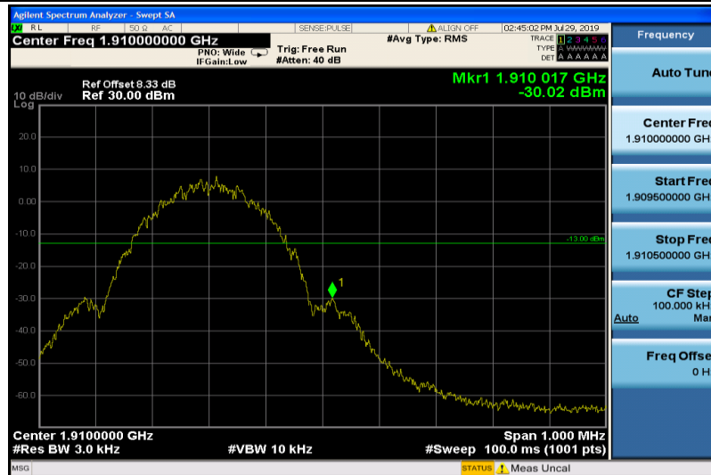
GPRS1900-810
