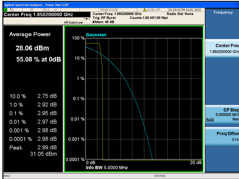
GPRS1900-512
