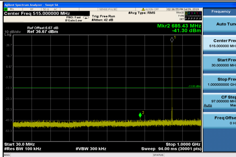
EGPRS850-251-30~1000
