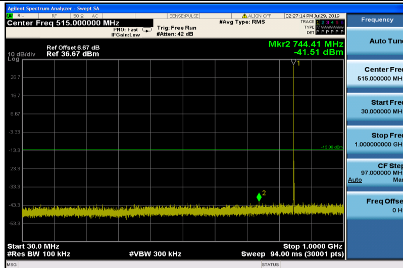
GSM850-251-30~1000
