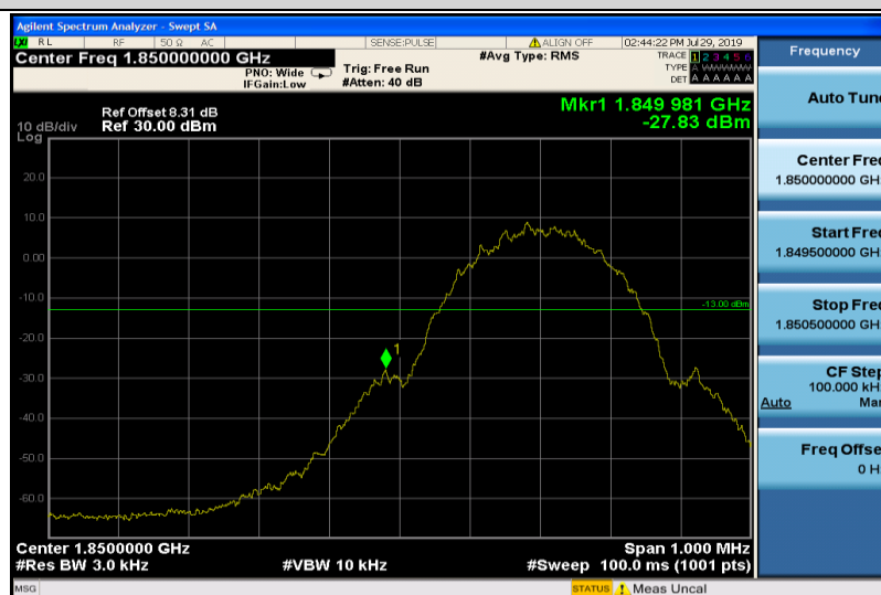
GPRS1900-512
