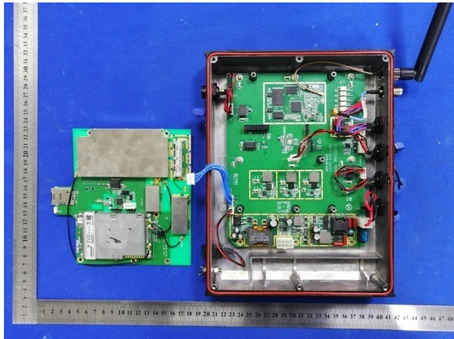
EUT Photo 10
