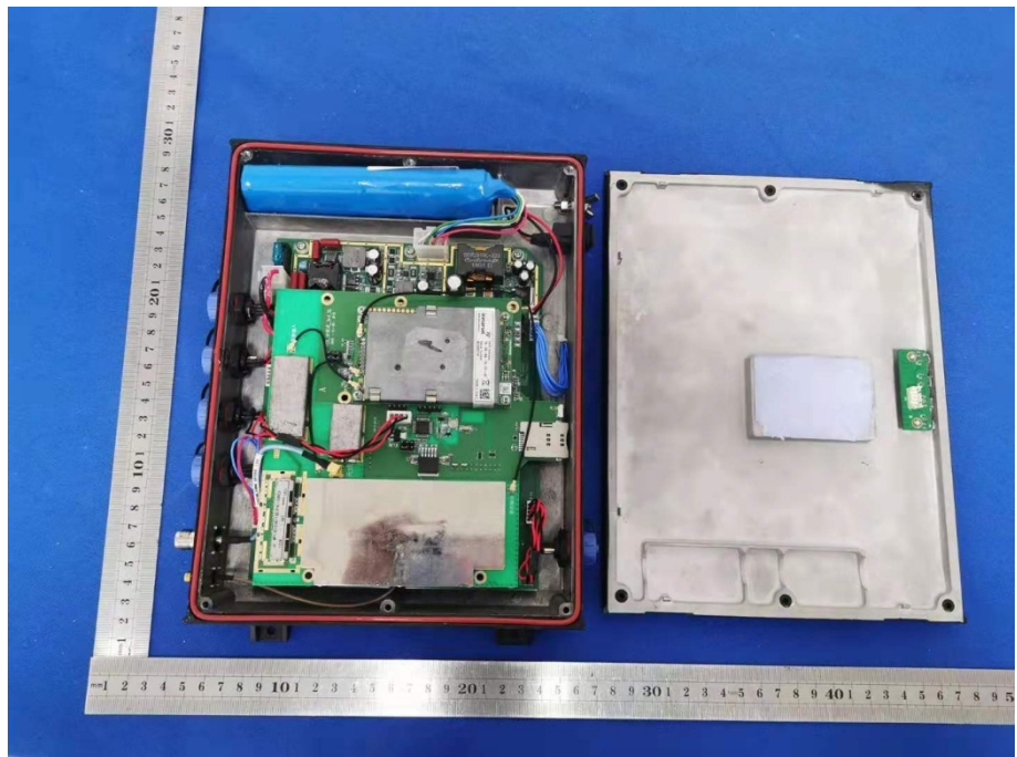
EUT Photo 8
