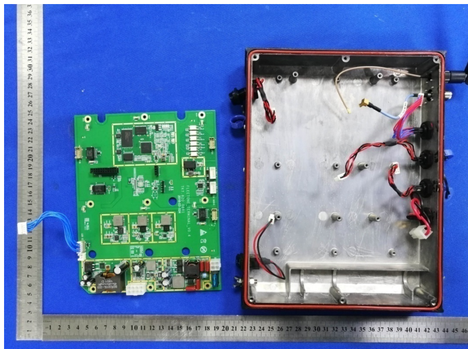
EUT Photo 11
