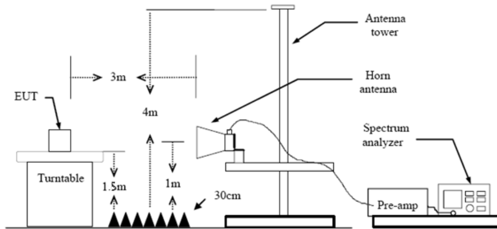
1000MHz Test Setup
