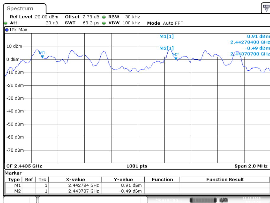
CFS NVNT GFSK 2443MHz Ant1
