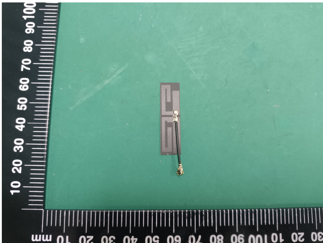
BLE Antenna
