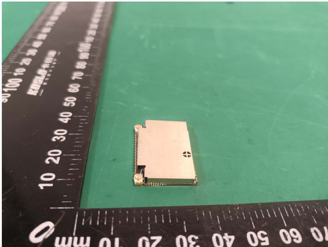
LoRa Antenna 1
