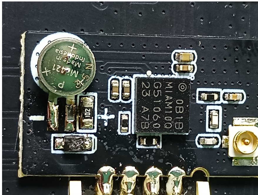
BLE/Wi-Fi ANT
