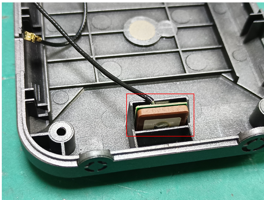
GPS ANT
