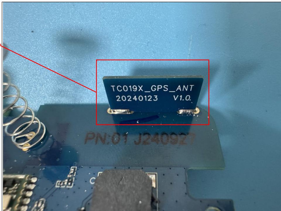
GNSS ANT
