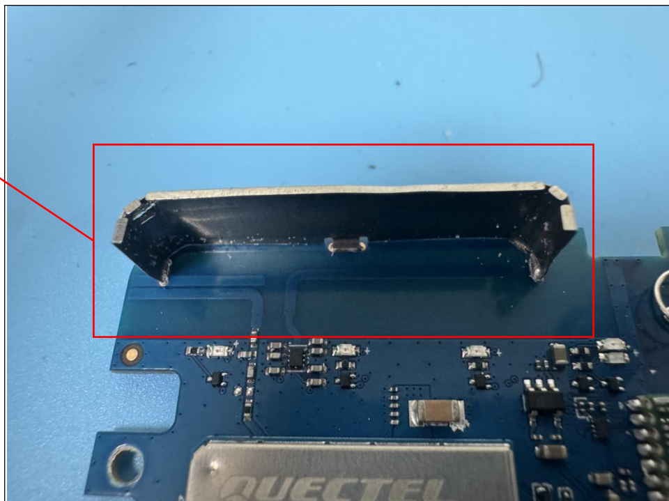
GSM/LTE ANT
