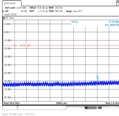
BLE_2M-Ant1-2402-30~1000-PASS
