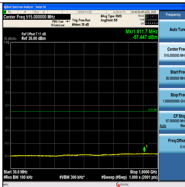
Band7 20MHz QPSK 21100 1RB#0 30~1000 30~1000
