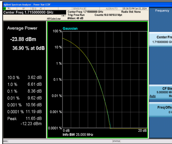
Band4-10MHz-QPSK-20000-1RB#0-PASS
