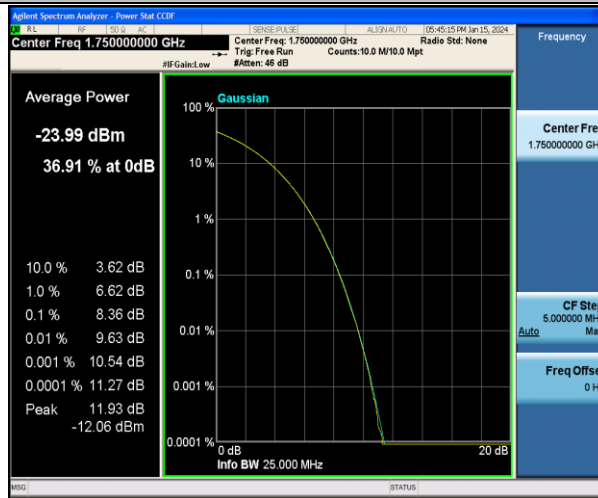
Band4-10MHz-QPSK-20350-1RB#0-PASS
