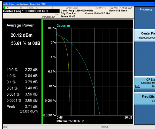
Band2-10MHz-QPSK-18900-1RB#0-PASS
