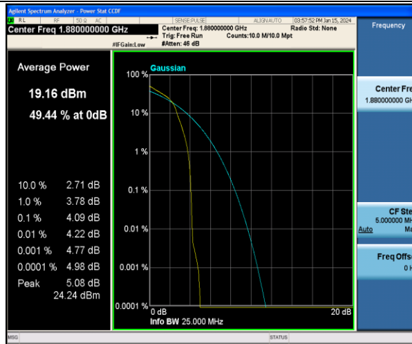
Band2-20MHz-16QAM-18900-1RB#0-PASS
