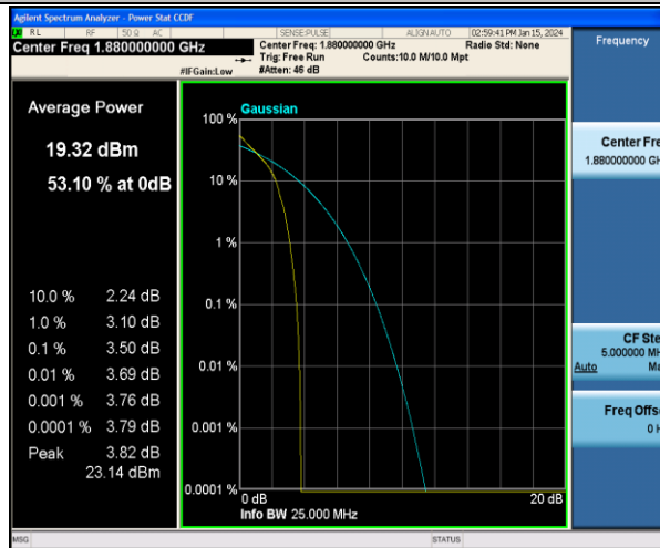
Band2-3MHz-QPSK-18900-1RB#0-PASS
