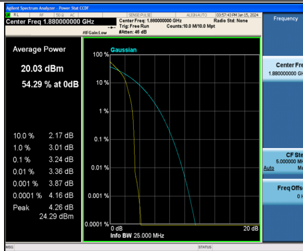
Band2-20MHz-QPSK-18900-1RB#0-PASS
