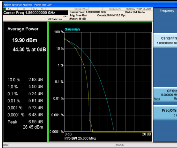
Band2-20MHz-QPSK-18700-1RB#0-PASS
