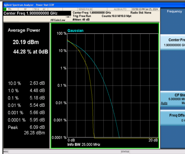
Band2-20MHz-QPSK-19100-1RB#0-PASS
