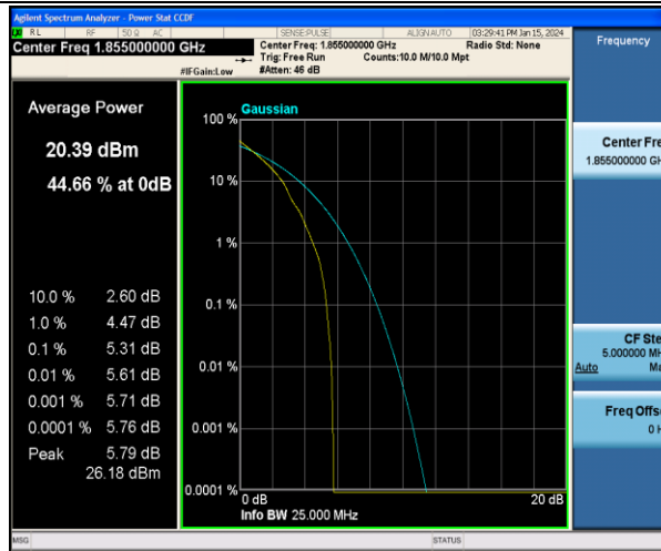
Band2-10MHz-QPSK-18650-1RB#0-PASS
