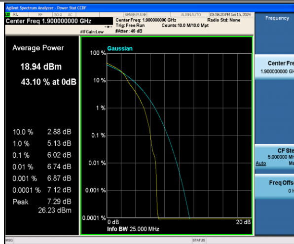
Band2-20MHz-16QAM-19100-1RB#0-PASS
