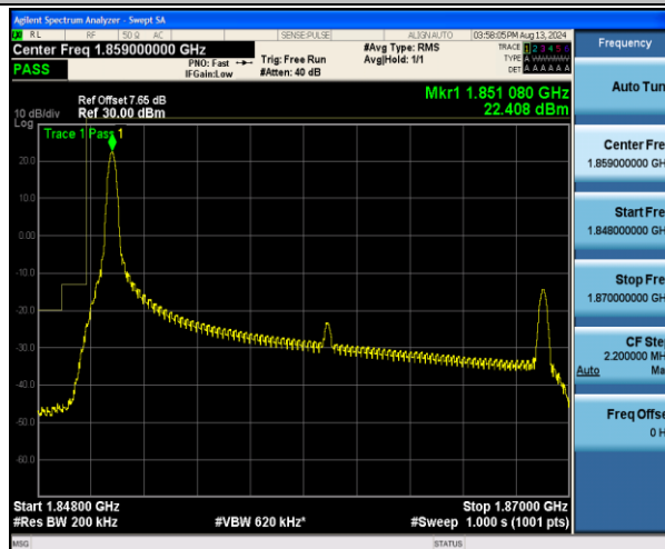
Band2 20MHz QPSK 18700 1RB#0
