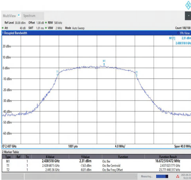
11G-Ant1-2437
