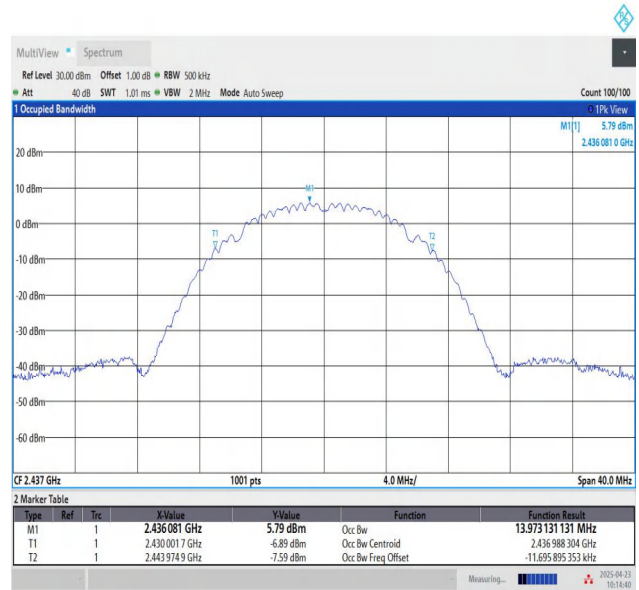
11B-Ant1-2437
