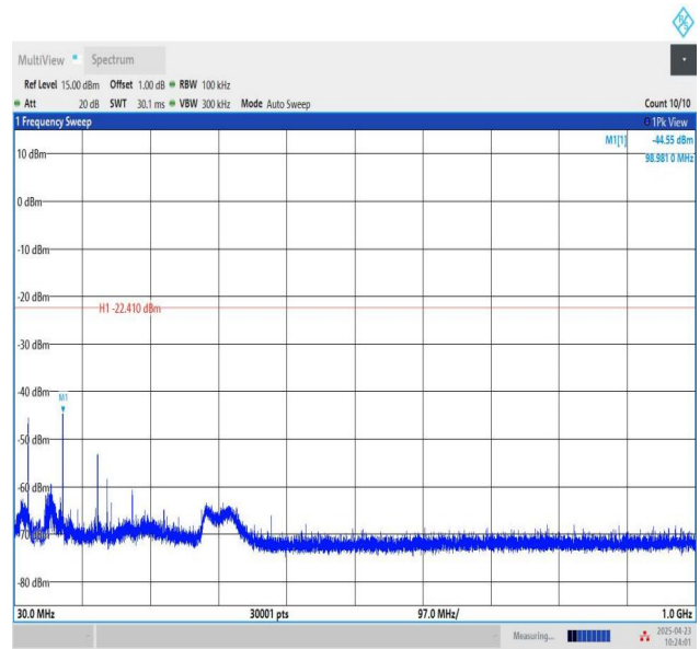
11G-Ant1-2437-30~1000-PASS
