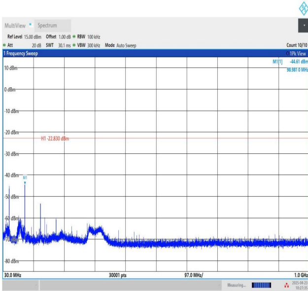
11G-Ant1-2462-30~1000-PASS
