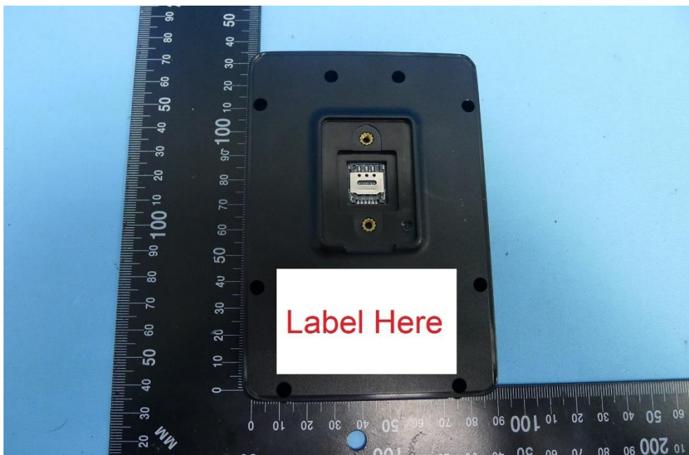
(8) EUT Photo
