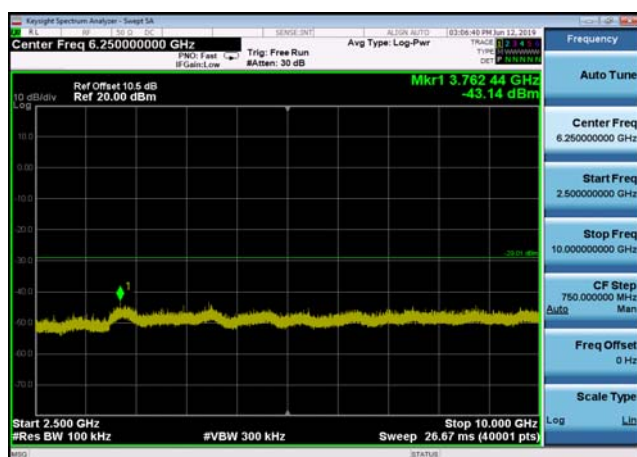
,Plot 4,2500MHz~10000MHz-802.11n(HT40 ) ,2452MHz,Ant0
