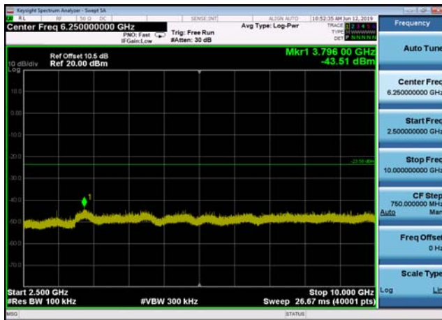
,Plot 4,2500MHz~10000MHz-802.11g ,2437MHz,Ant0
