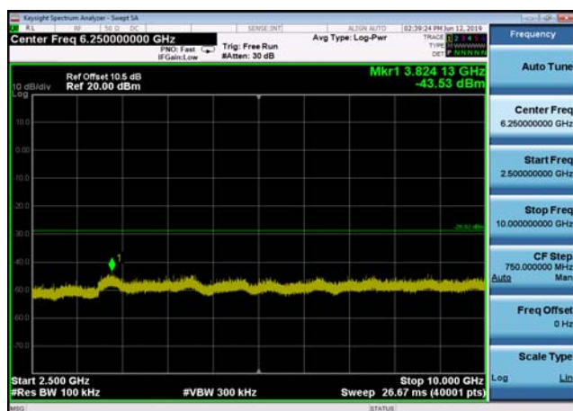
,Plot 4,2500MHz~10000MHz-802.11n(HT40 ) ,2437MHz,Ant0
