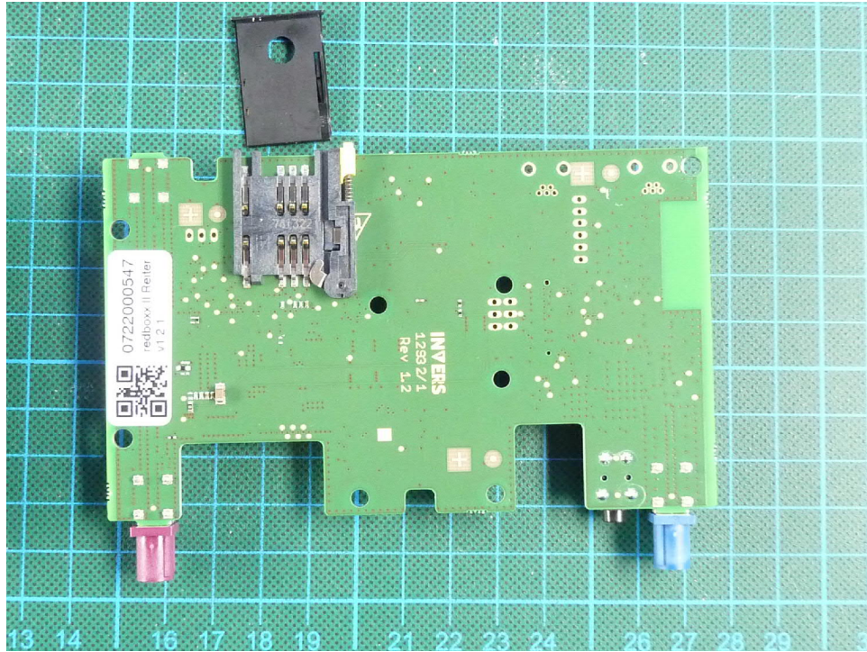
181948_eut18.JPG : EUT main unit PCB B bottom view
