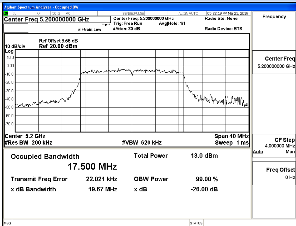
IEEE 802.11ac20 / Channel 40 / 5200MHz_Ant_4
