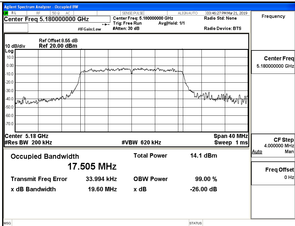
IEEE 802.11ac20 / Channel 36 / 5180MHz_Ant_3
