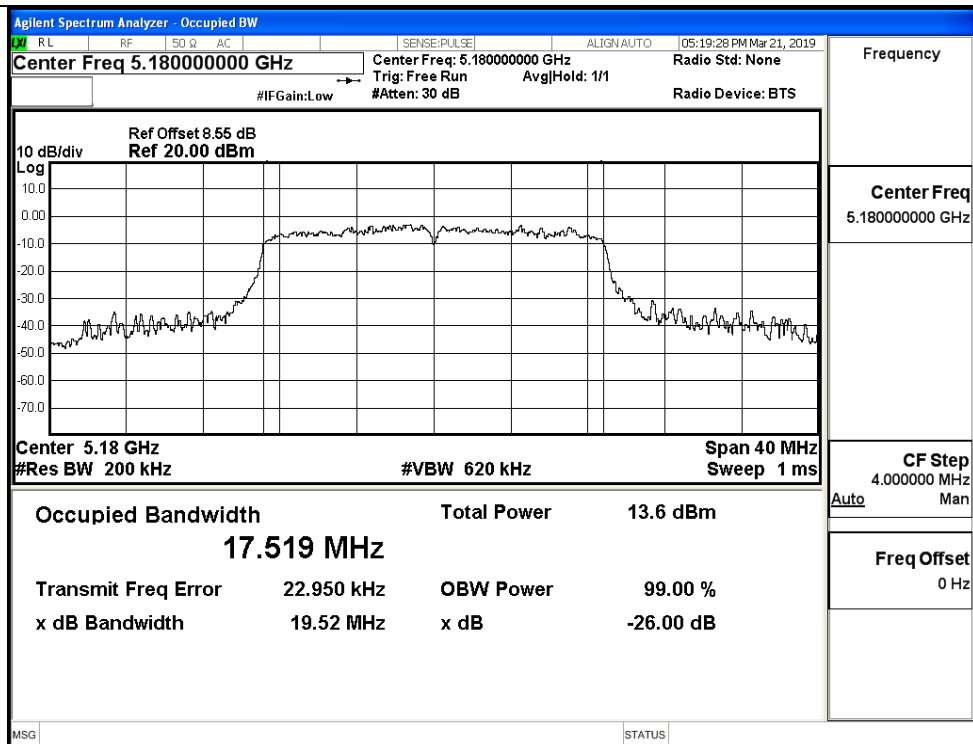
IEEE 802.11ac20 / Channel 36 / 5180MHz_Ant_4
