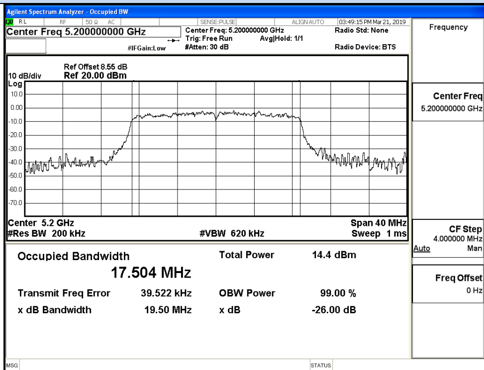
IEEE 802.11ac20 / Channel 40 / 5200MHz_Ant_3
