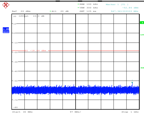
2DH5 ANT1 2441 30~1000
