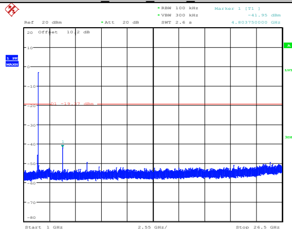
2DH5 ANT1 2402 1000~26500
