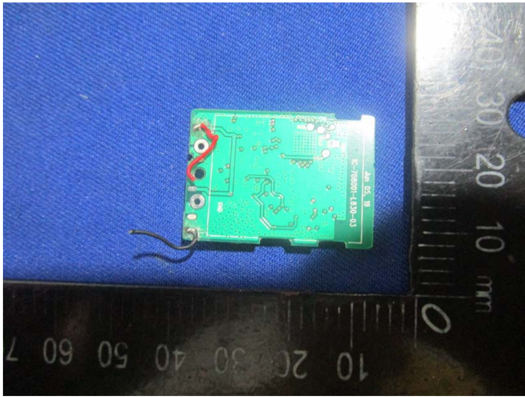
RF ANT
