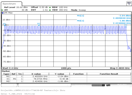
GFSK_Hopping_DH1
