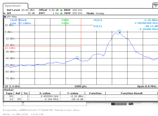
GFSK_Low_DH1
