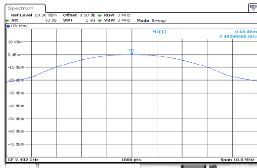
GFSK_Low_DH1
