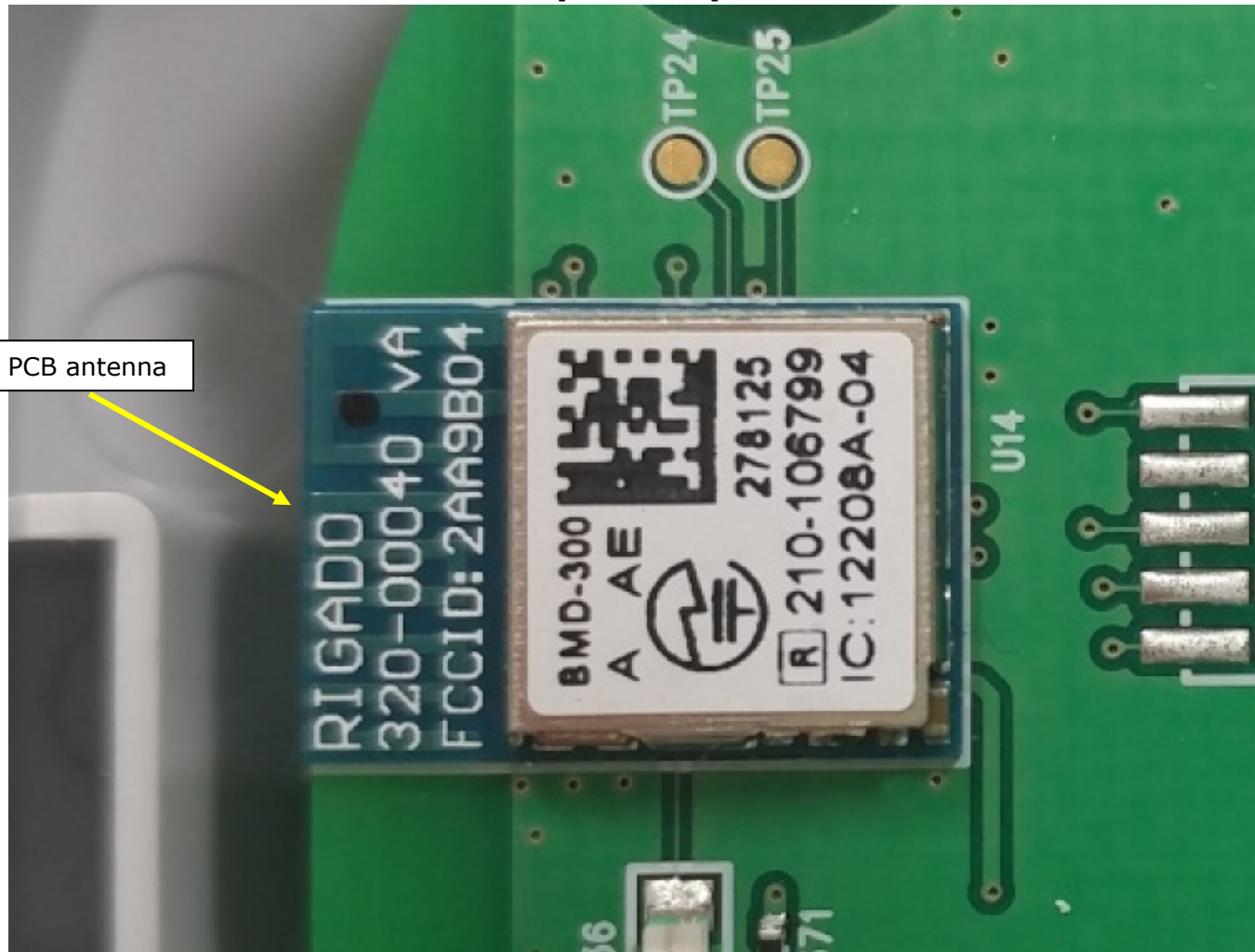
[DXX module]
