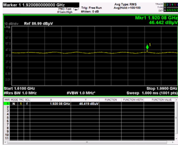
Horizontal(1 610-1 990 MHz)
