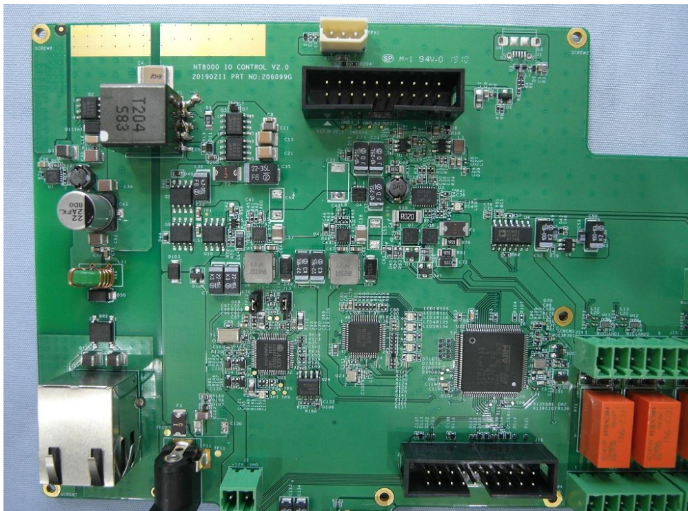
(44) EUT Photo
