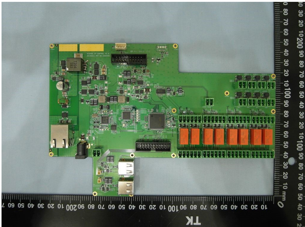
(44) EUT Photo
