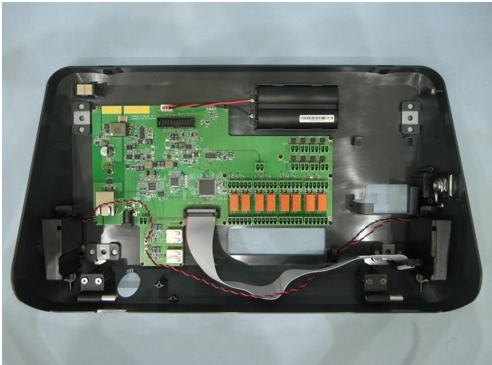
(40) EUT Photo
