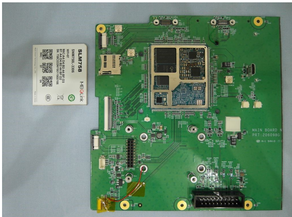
(30) EUT Photo
