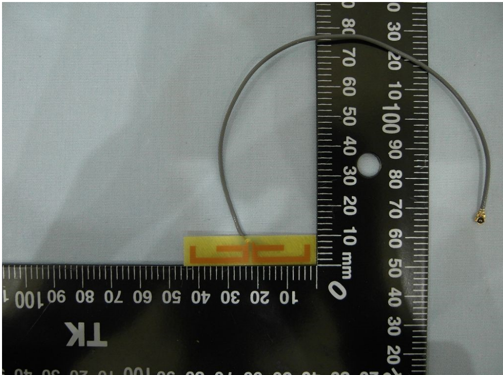
(36) EUT Photo
