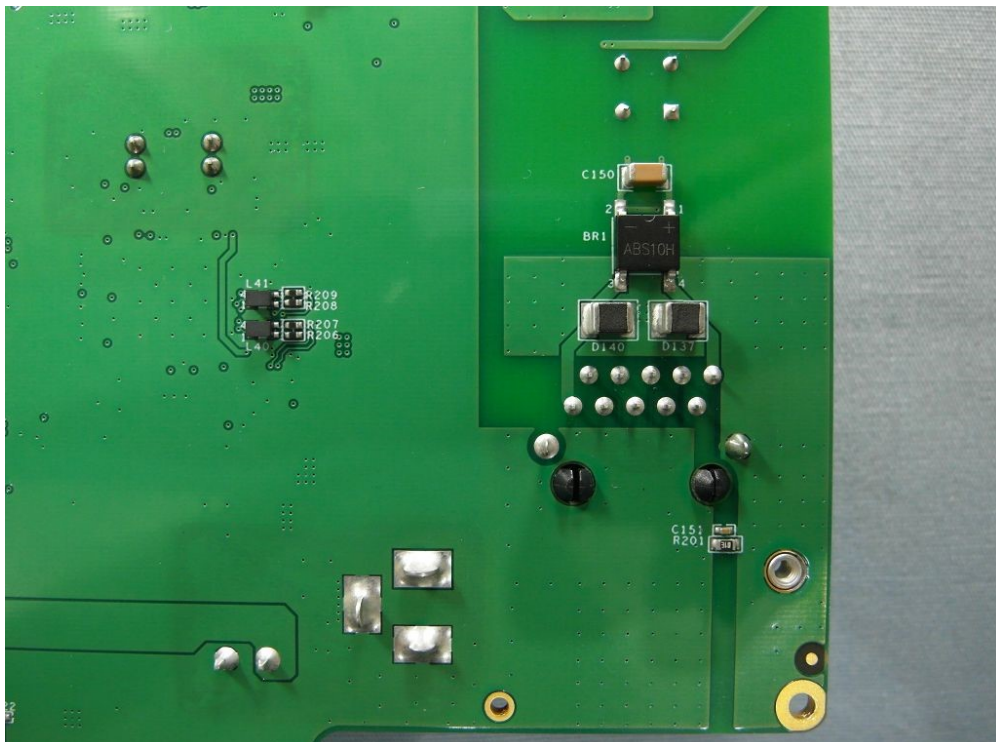
(47) EUT Photo
