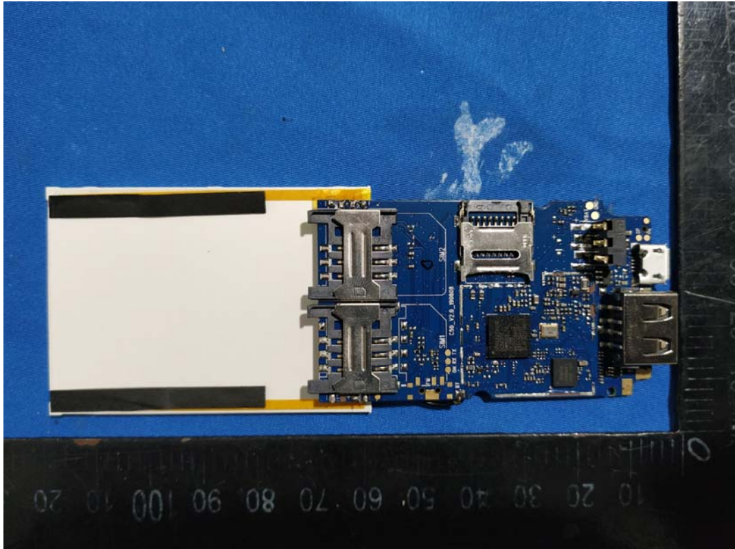
GSM ANT
