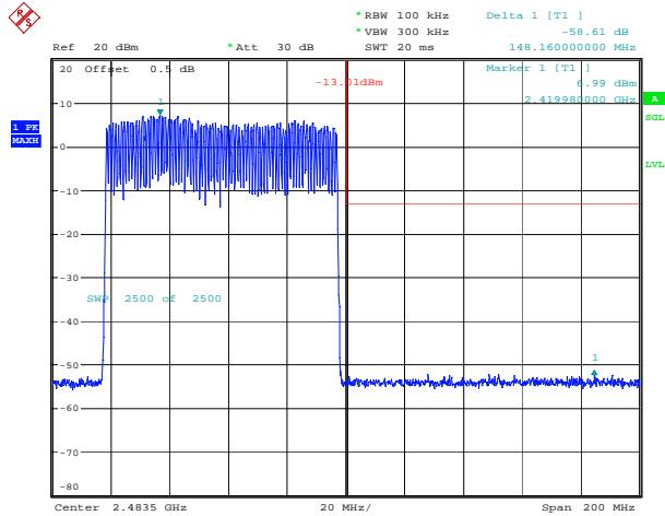
DH1_Hopping_Upper
