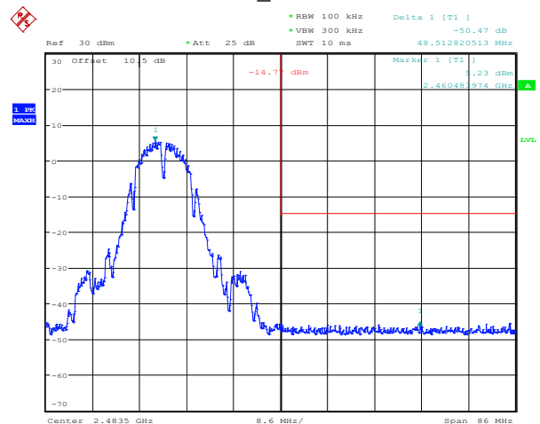
802.11b_2462MHz
