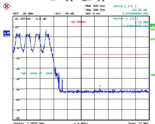
DH1_Hopping_Upper 53.36dB
