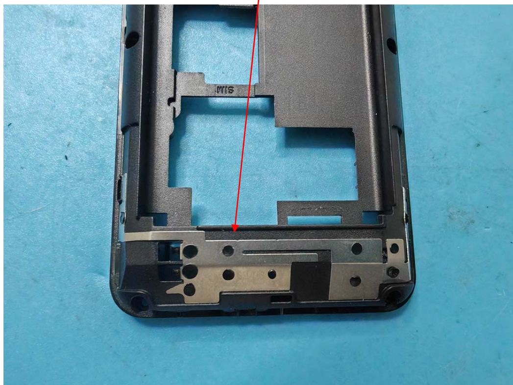
GSM Antenna
